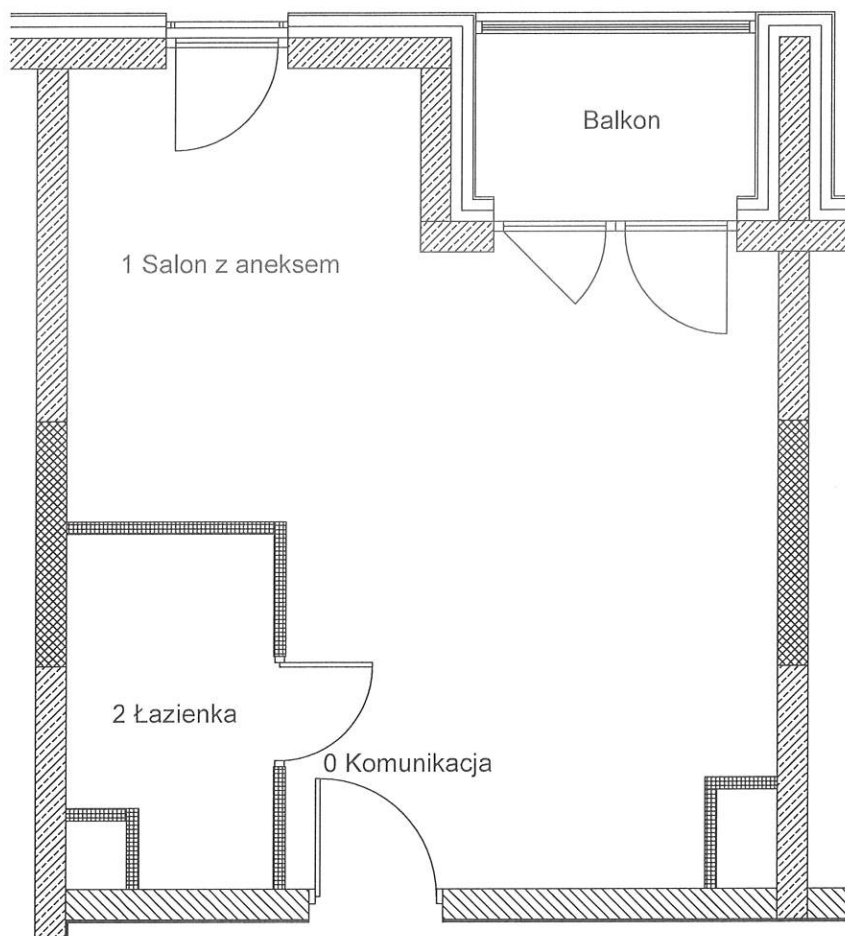
RZUT LOKALU
