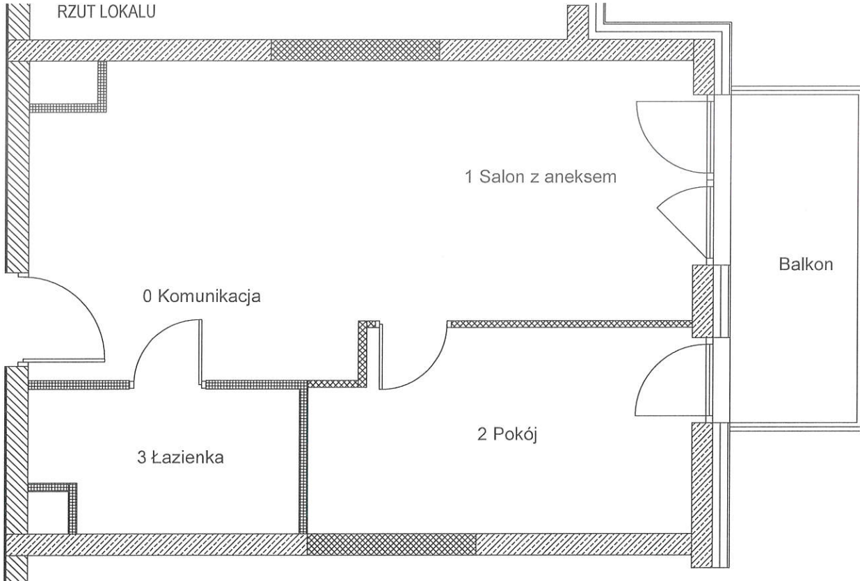
RZUT LOKALU
